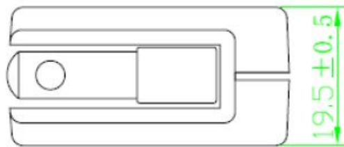
俯视图
